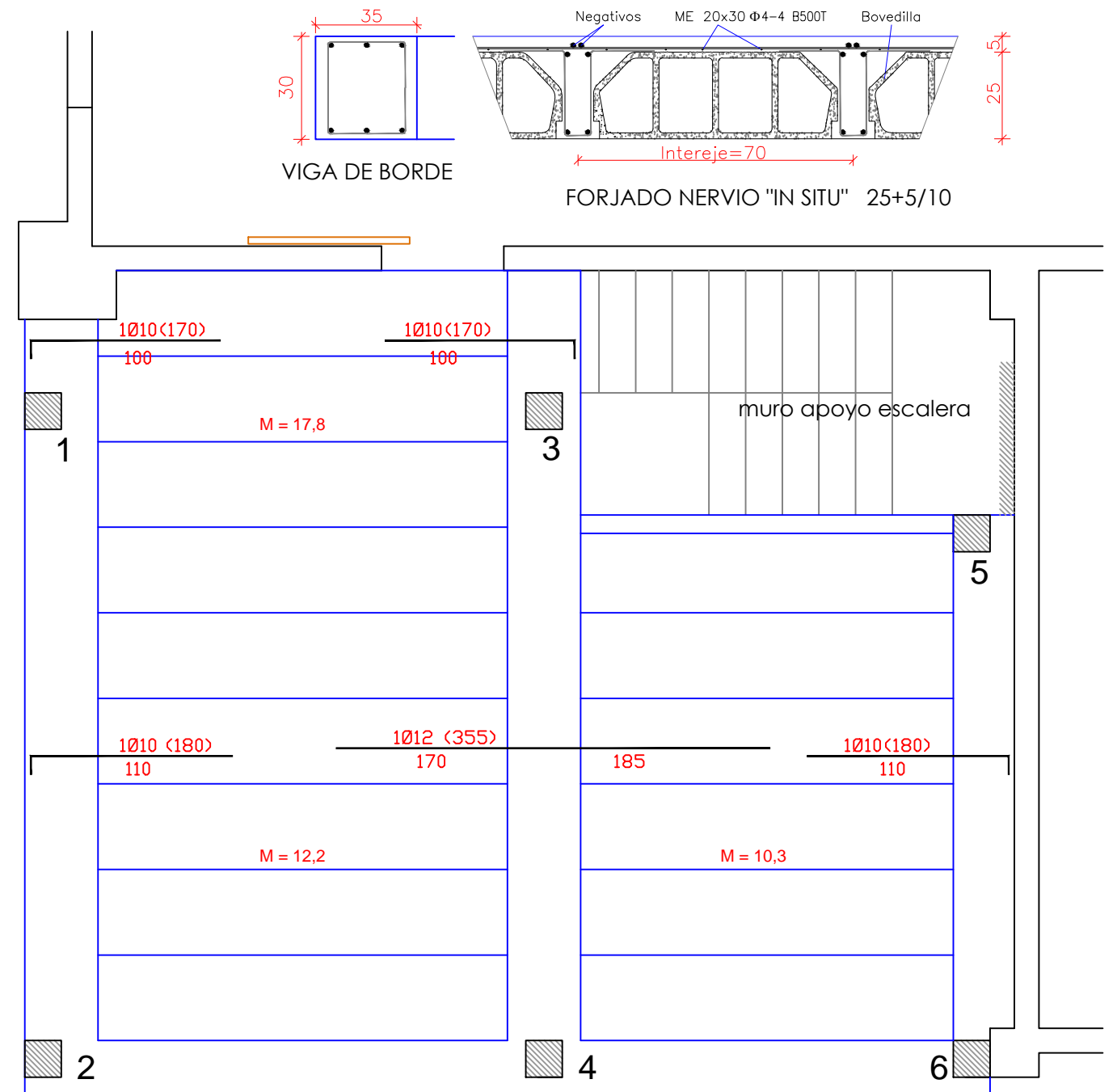
FORJADO DE PLANTA 1
